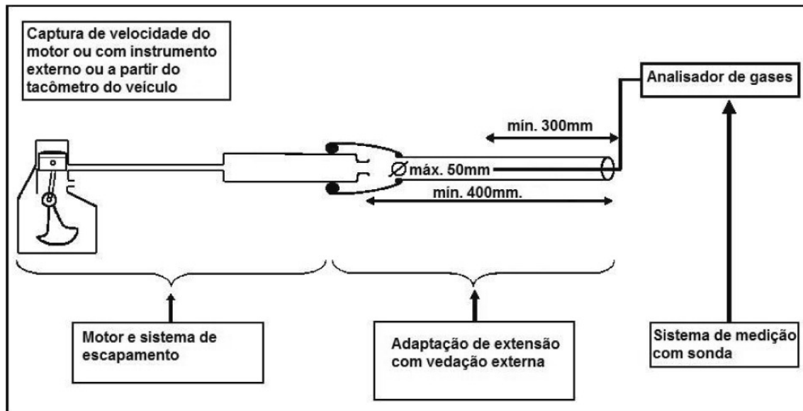
Figura 1 - Adaptador externo com coifa flexível
