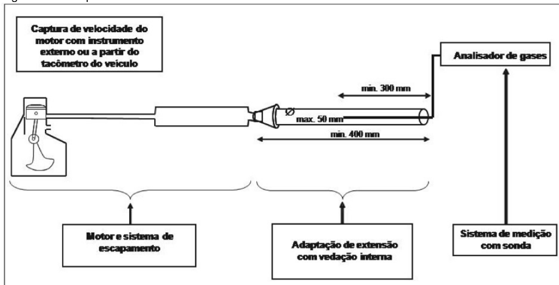
Figura 3 - Adaptador interno
